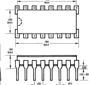
16-Pin Cavity Dual-In-Line Package (D)
