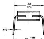
16-Pin Cavity Dual-In-Line Package (D)
