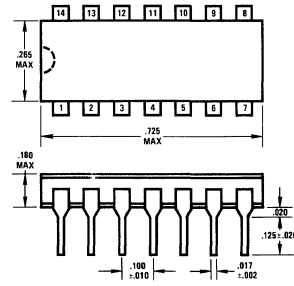
14-Pin Cavity Dual-In-Line Package (D)
