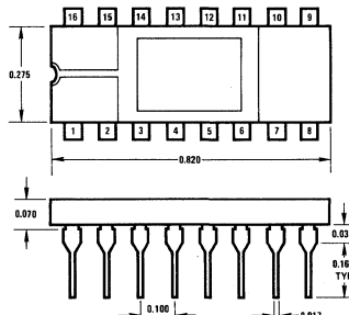
16-Pin Cavity Dual-In-Line Package (D)
