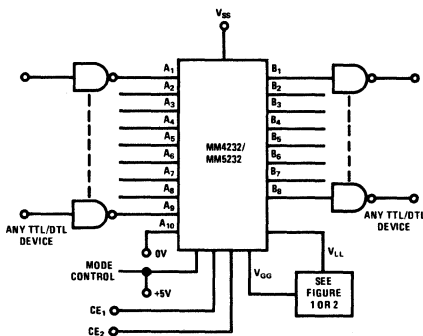
TTL/MOS Interface
