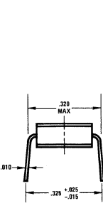
14-Pin Cavity Dual-In-Line Package (D)
