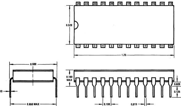
24-Pin Cavity Dual-In-Line Package (D)
